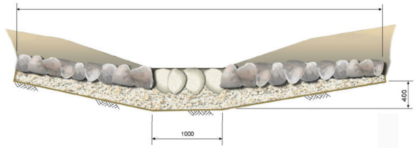
SECTION 4 N.T.S.
